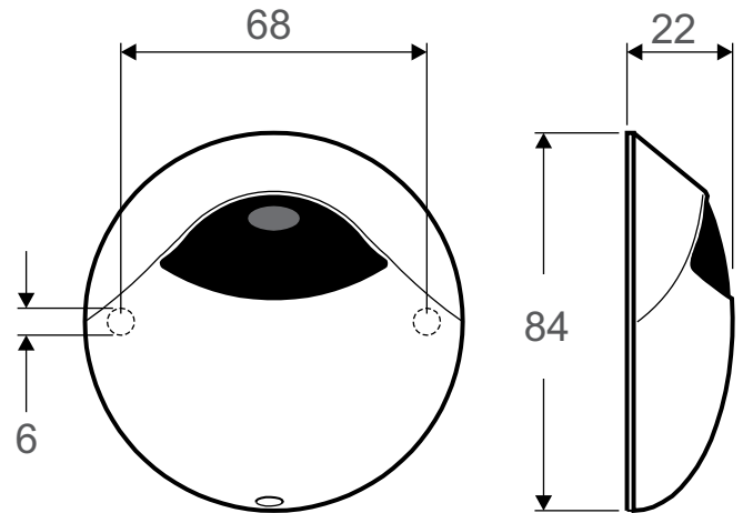
Rada 122 Sensor
